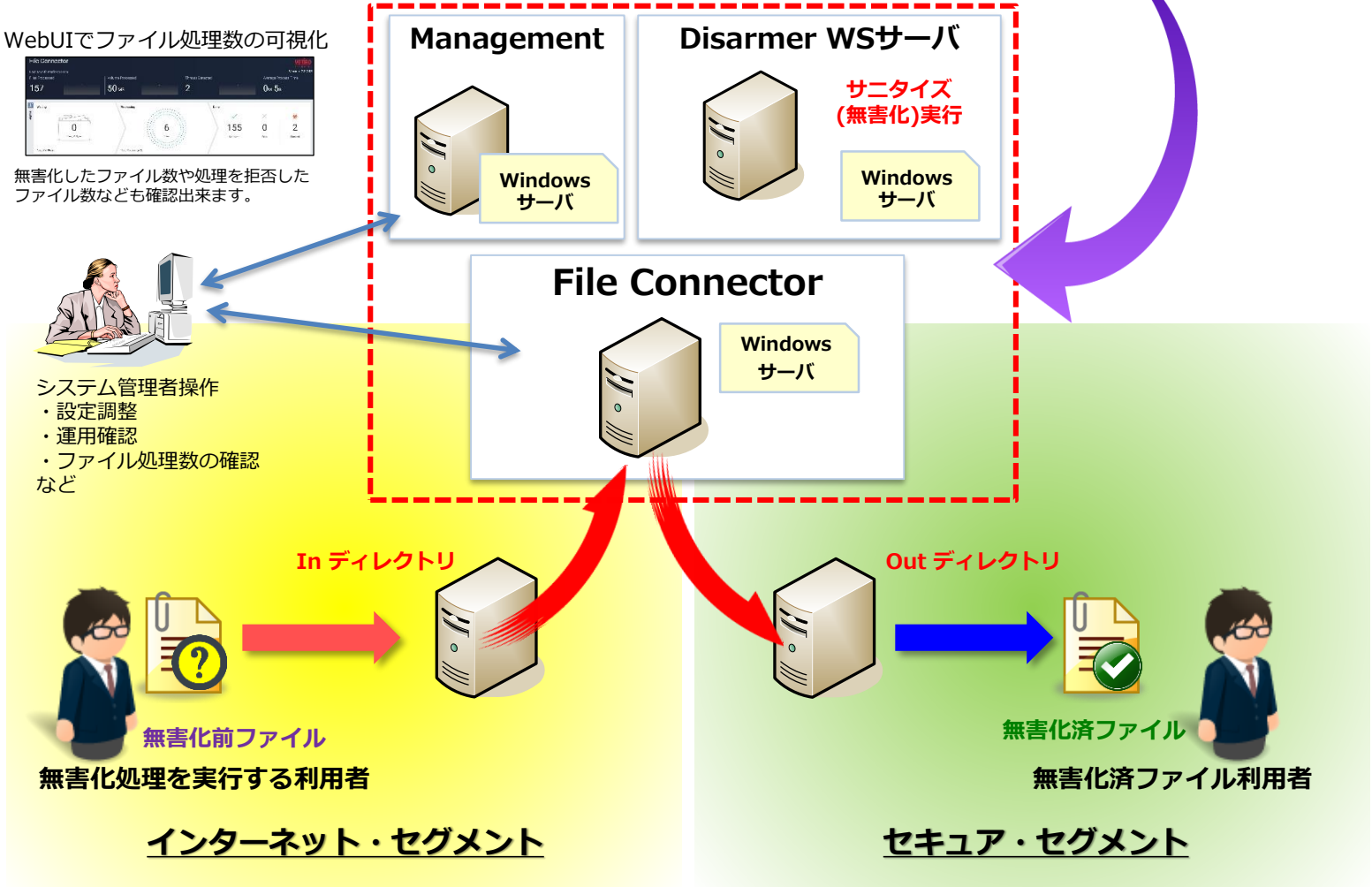
Votiro Disarmer FC アプライアンスサーバ構成概要
